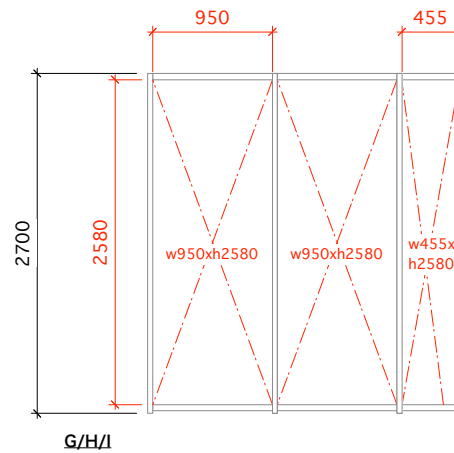
台灣館內攤位隔板尺寸
